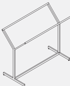
ケースWハンガー RIALW-14R W1200 D550 H1000 スチール・Crメッキ / 焼付塗装(白)
