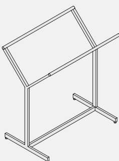
ケースWハンガー RIALW-14L W900 D550 H1000 スチール・Crメッキ / 焼付塗装(白)
