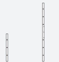
フレームパイプ白 (H550用) ACTW-PA066E W30 D30 H490 フレームパイプ白 (H1100用) ACTW-PA066N W30 D30 H1040 フレームパイプ白 (H1650用) ACTW-PA066T W30 D30 H1590 フレームパイプ白 (H2200用) ACTW-PA066Z W30 D30 H2140
