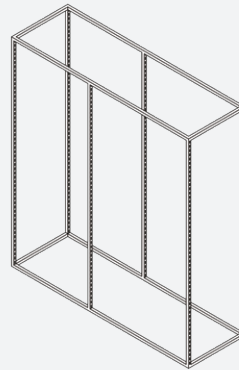
本体フレーム INTI-23W W1206 D382 H1350
