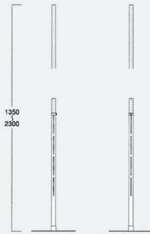
本体ポール FD073 (CORE) スチール・CrHL仕上げ
