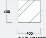
ガラス AR098DD (NNB) 透明ガラス8t
