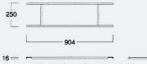
棚受け渡し (W900) BC042KY (NN) スチール・Crメッキ
