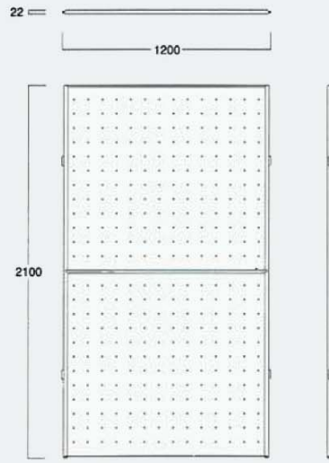
アルミパネル RL090PX (CORE) スチール・CrHL仕上げ/アルミ・アルマイト仕上げ
