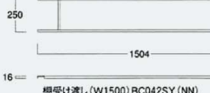
棚受け渡し (W1500) BC042SY (NN) スチール・Crメッキ
