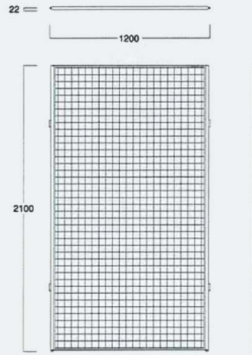
メッシュパネル RH090PX (CORE) スチール・CrHL仕上げ/スチール50ピッチメッシュ・Crメッキ
