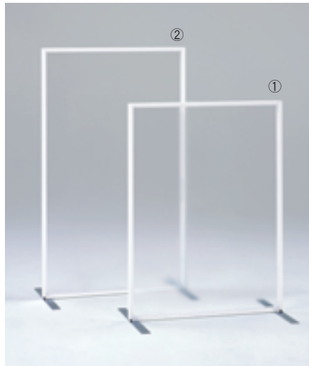
① MODEL-17 W900 D550 H1200 本体 アルミ・焼付塗装(白)・アクリル3t(タベストリー) ② MODEL-18 W900 D550 H1500 本体 アルミ・焼付塗装(白)・アクリル3t(タベストリー)
