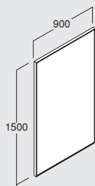
本体パネル (H1500) EQ051KS アルミ・焼付塗装(白) /PET-G樹脂(スモークブラウン)
