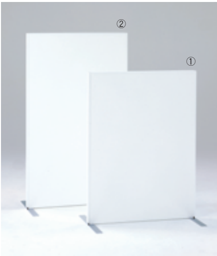
① MODEL-15 W900 D550 H1200 本体 アルミ・焼付塗装(白)・ペーパーハニカム ② MODEL-16 W900 D550 H1500 本体 アルミ・焼付塗装(白)・ペーパーハニカム
