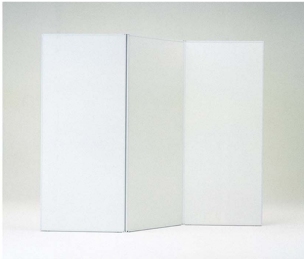
MODEL-5 本体パネル アルミ・焼付塗装(白)・ペーパーハニカム W2544 D390 H2100
