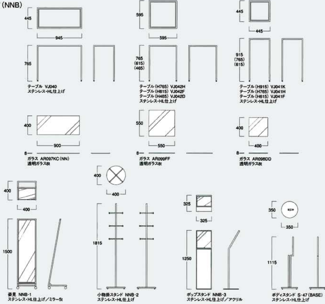
NNB-3 本体 ステンレス・HL仕上げ/ 板面 表・透明アクリル3t 裏・乳半アクリル5t W325 D325 H1250
