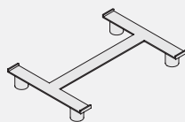
脚 LJ-VC056G W665 D467 H85 スチール・Crメッキ
