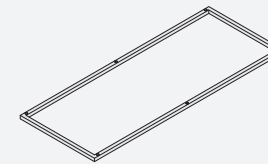
ガラス棚受け RIALS-BB142LC (黒) RIALS-BE142LC (古美色) W1016 D400 H16
