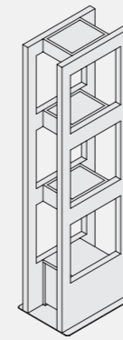
本体 NEST-12 (白) NEST-13 (チーク) NEST-14 (マホガニー) W600 D450 H2050 SUS・HL 仕上げ / LED 照明
