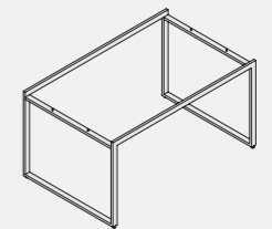
テーブル脚 NEST-VJ055RJ W1340 D840 H700 SUS・HL 仕上げ
