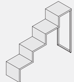
本体 NEST-15 (白) NEST-16 (チーク) NEST-17 (マホガニー) W450 D1800 H1300 SUS・HL 仕上げ
