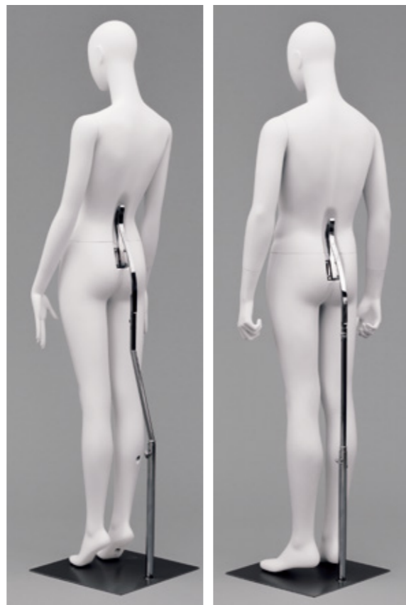
WAIST STAND Base:BIT1.2.3 Aタイプ(B-10 / S-73) BITM1 Cタイプ(B-10 / S-75) BITM2.M3 Aタイプ(B-10 / S-73)
